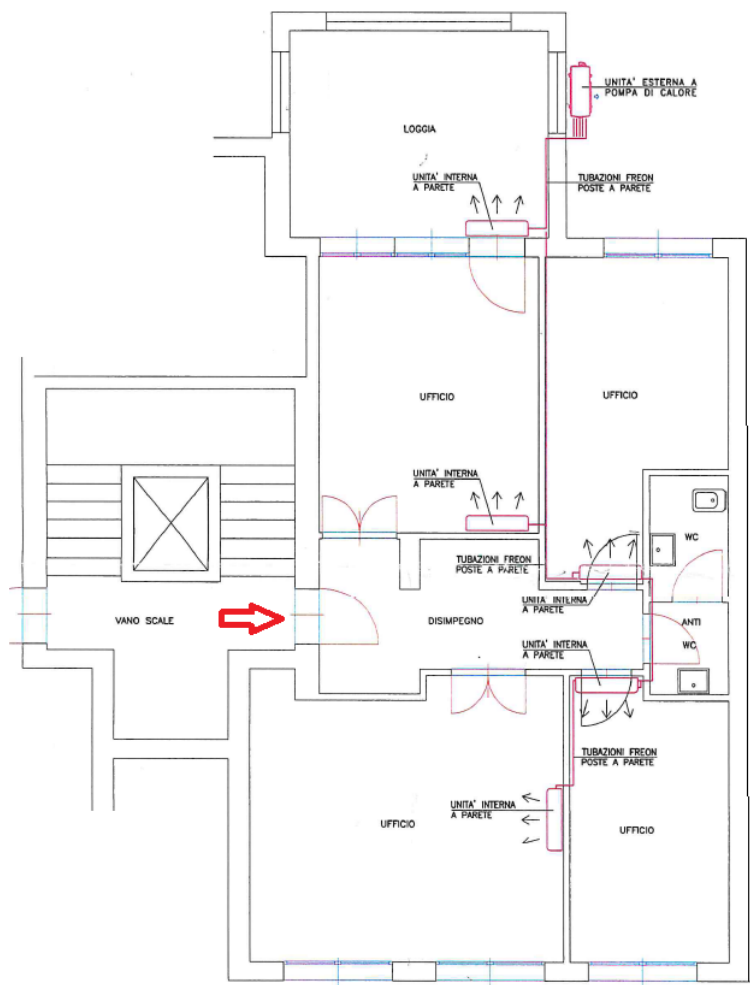
PIANO SECONDO
