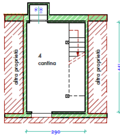
Pianta interrato
