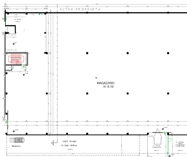
PIANO TERRA-RIALZATO
