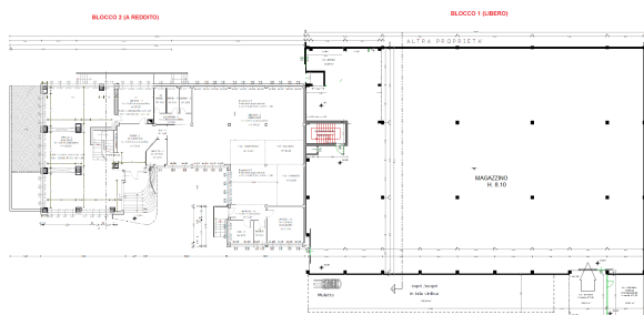
PIANO TERRA-RAZZATO
