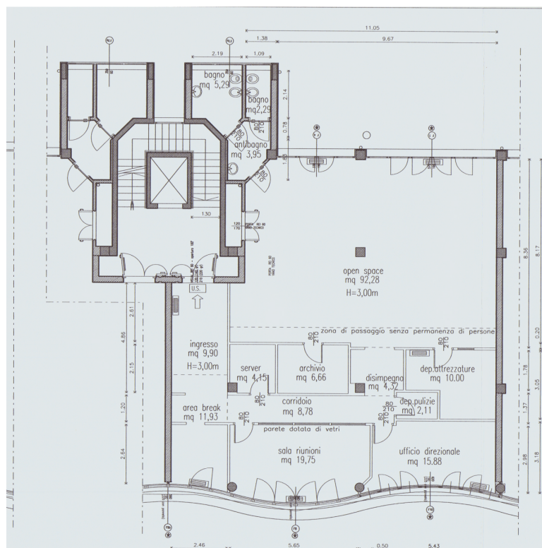
PIANO PRIMO
