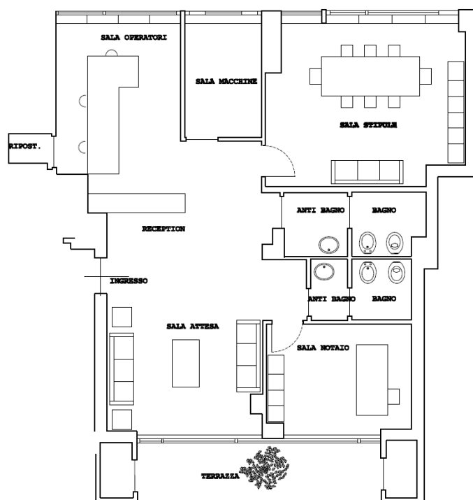
PIANO PRIMO
